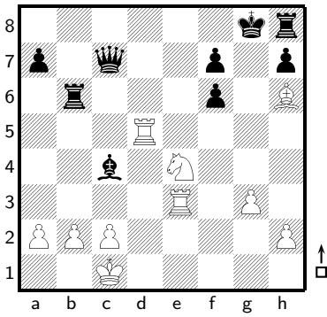
No. 669 白先
