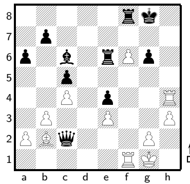
No. 672 白先
