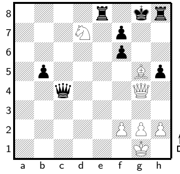
No. 671 白先
