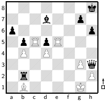
No. 668 白先
