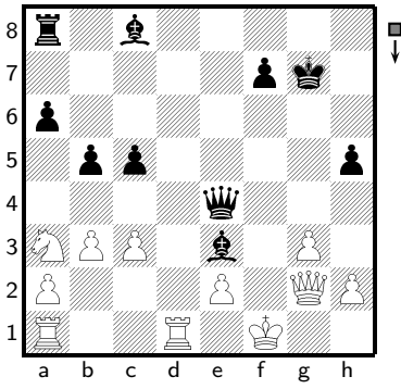
No. 4442 黑先
