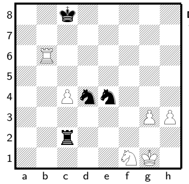
No. 4446 黑先
