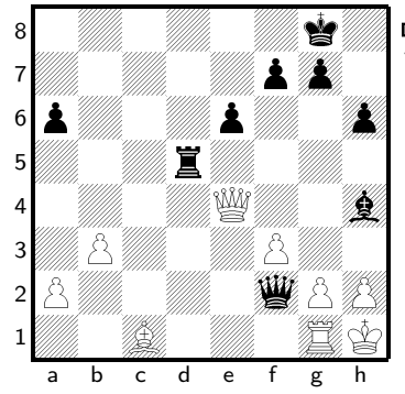
No. 4445 黑先
