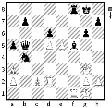
No. 4443 黑先
